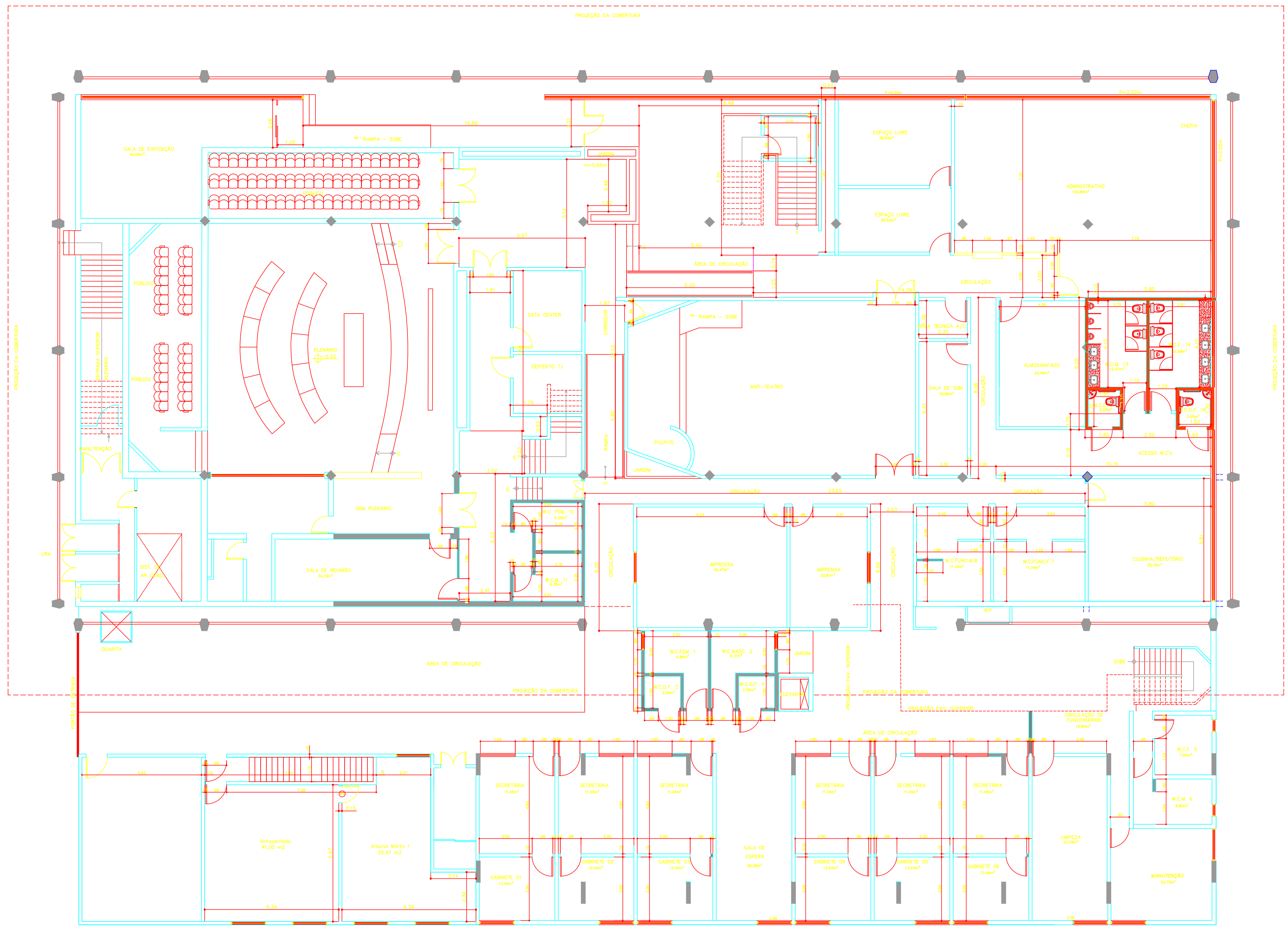
PAVIMENTO TÉRREO esc. 1:100
